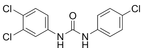
Triclocarban
